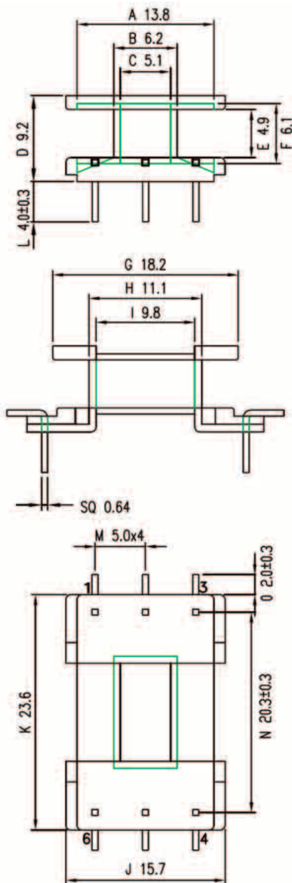
TPI-0501907(V) - каркас 1 секция 6 выводов (EI-19-10-6PIN)
