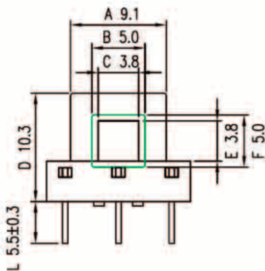
TPI-0501304(H) - каркас 1 секция 5 выводов (EE-13-3.8/28x29-5PIN)
