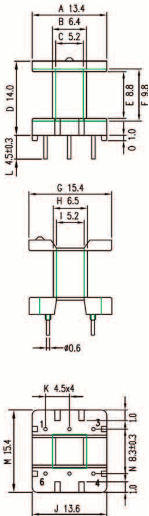
TPI-0501906(V) - каркас 1 секция 6 выводов (EI-19-5-6PIN)
