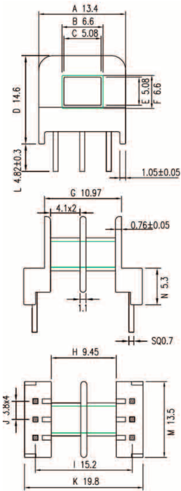
ТPI-0501910(H) - каркас 2 секции 6 выводов (EE-19-6PIN)
