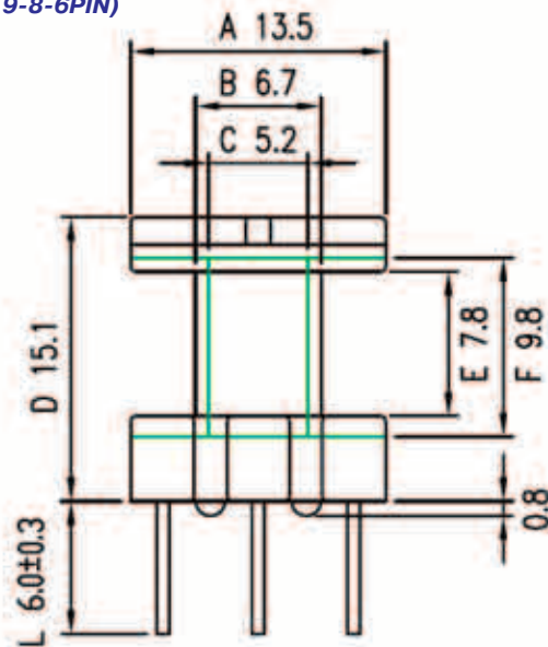
TPI-0501901(V) - каркас 1 секция 6 выводов (EI-19-8-6PIN)
