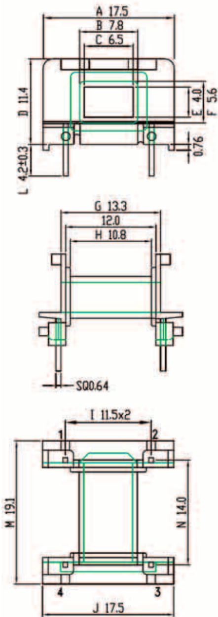
TPI-0501614(H) - каркас 1 секция 4 вывода (EE-16-4-4PIN)
