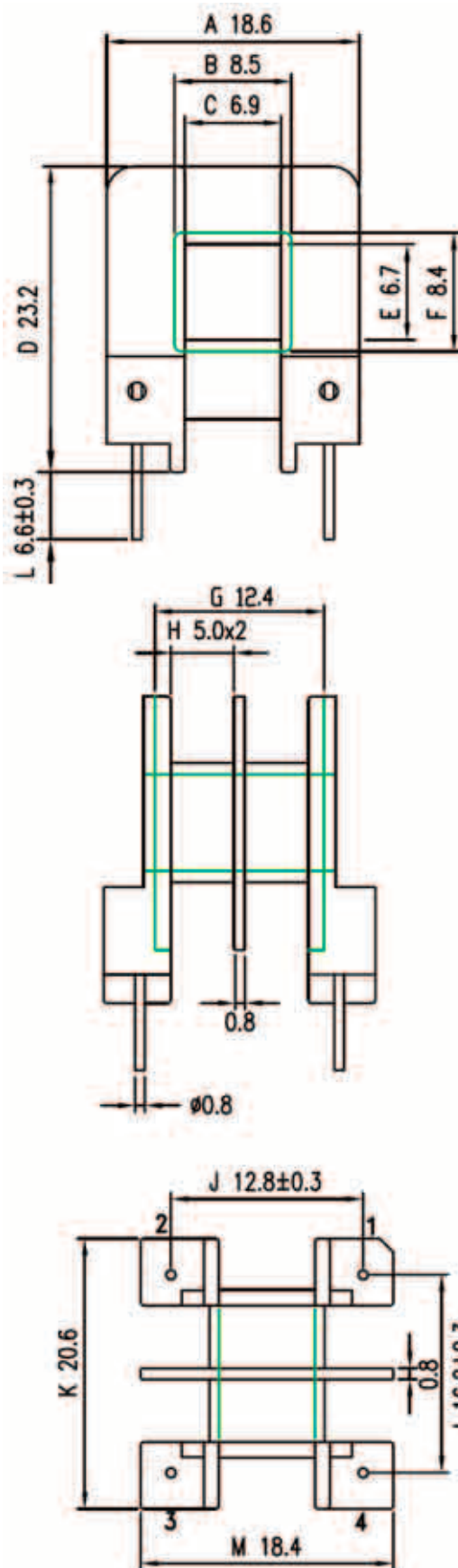
TPI-0502503(H) - каркас 1 секция 6 выводов (EE-25-19-4PIN)
