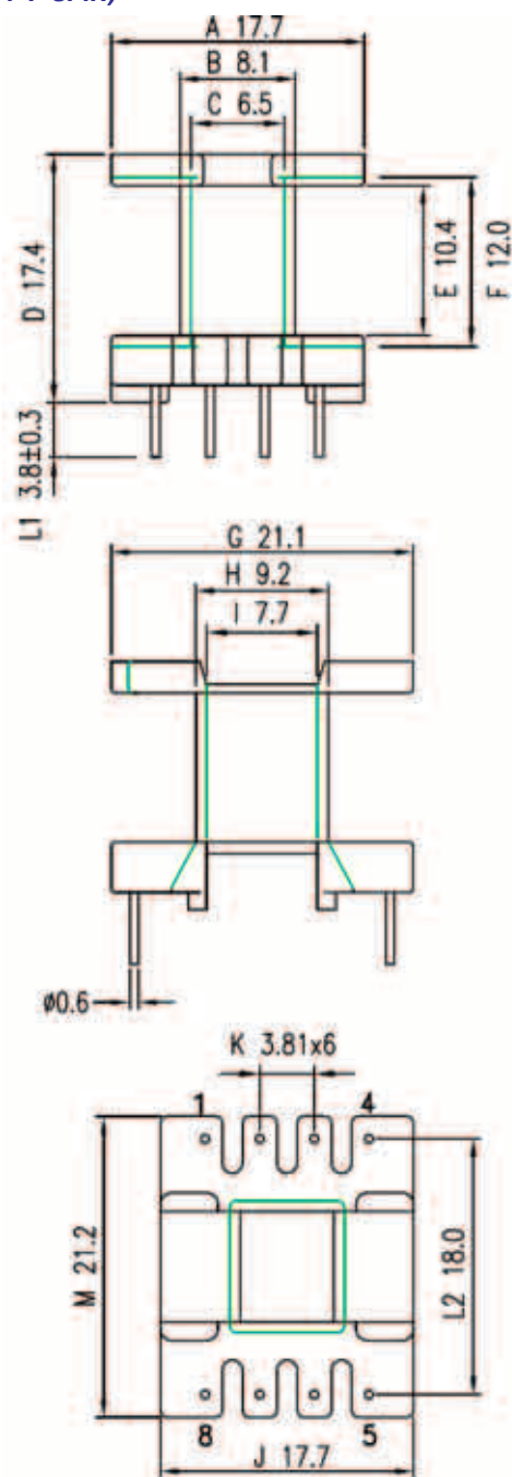
TPI-0502405(V) - каркас 1 секция 8 выводов (EI-24-7-8PIN)
