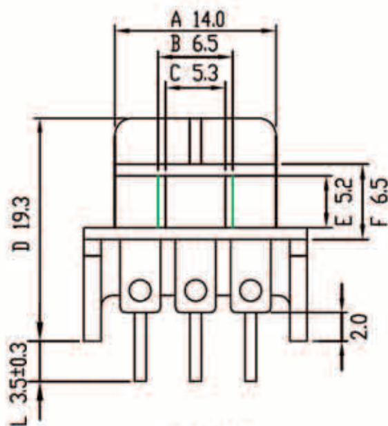
TPI-0502103(H) - каркас 2 секции 6 выводов (EI-21-5-3-6PIN)
