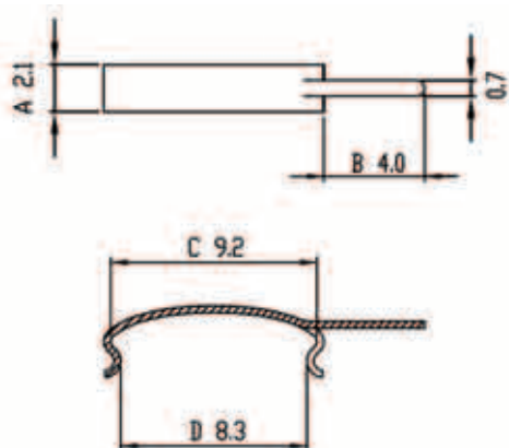
TPI-0503000-1(V) - скоба (EE-30-CLIP)
