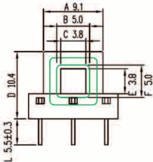
TPI-0501305(H) - каркас 1 секция 5 выводов (EE-13-3.8/28x29-5PIN)
