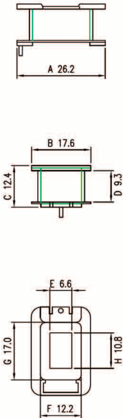
TPI-0502402(V) - каркас 1 секция (EI-24-10B)
