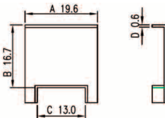
TPI-0502812(V) - каркас 1 секция (EI-28-12C)
