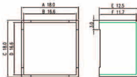
TPI-0501606(V) - каркас 1 секция 6 выводов (EE-16-6PIN-1SEC)
