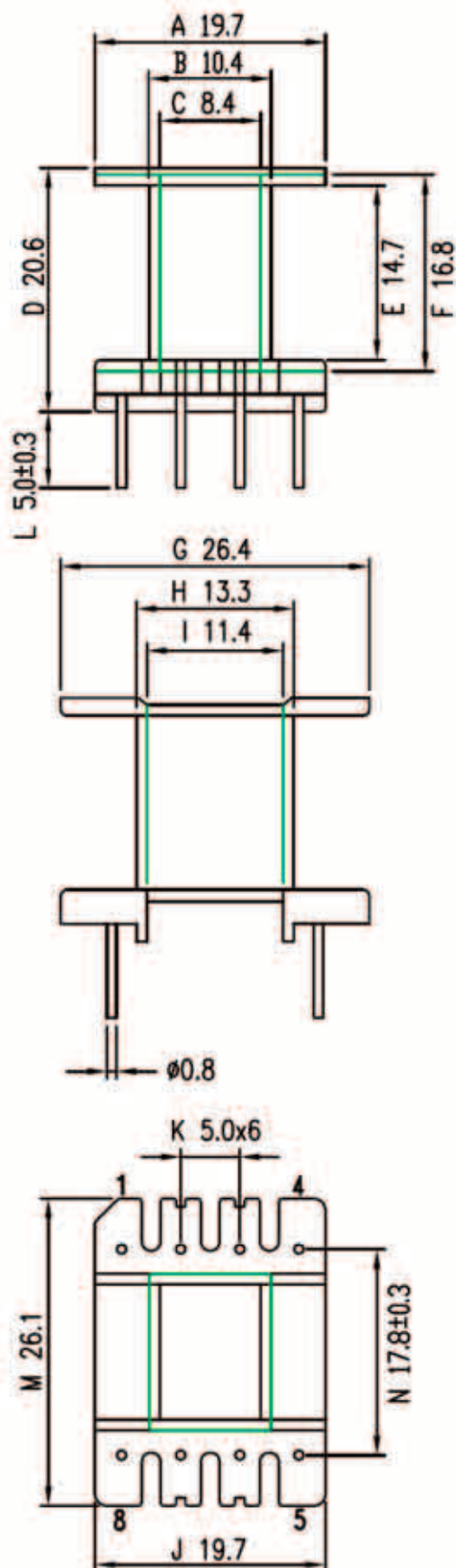
TPI-0502802(V) - каркас 1 секция 8 выводов (EI-28-11.5-8PIN)
