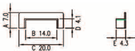
TPI-0502806-1(V) - каркас 1/2 секции (EI-28-12.5C)
