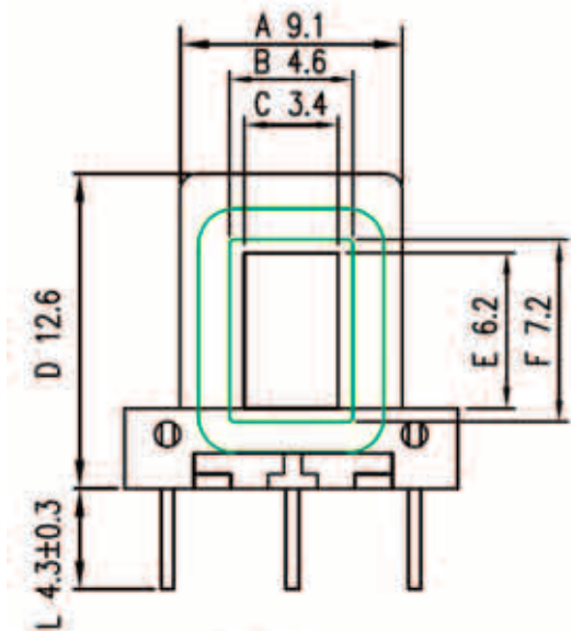
TPI-0501303(H) - каркас 1 секция 5 выводов (EE-13-6.1/28x29-5PIN)
