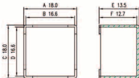
TPI-0501609 - крышка (EE-16-CASE, BOSS)
