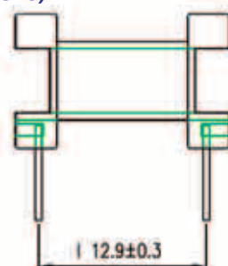
TPI-0501607(V) - каркас 2 секции 6 выводов (EE-16-6PIN-2SEC)
