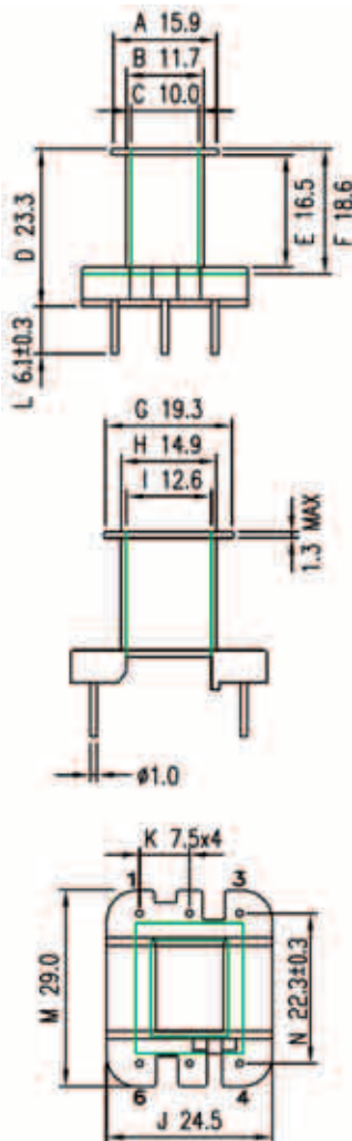
TPI-0503501(V) каркас 1 секция 6 выводов (EI-35-13-6PIN)
