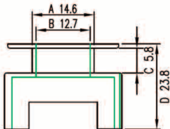
TPI-0502811(V) - каркас 1 секция (EI-28-12B)
