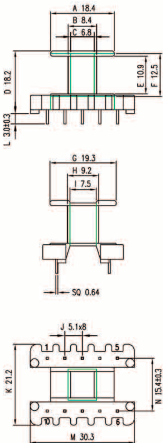
TPI-0502801(V) - каркас 1 секция 6 выводов (EI-28-11-6PIN)
