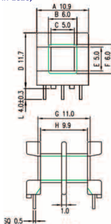
TPI-0501610(H) - каркас 2 секции 6 выводов (EE-16-6PIN-2SEC)
