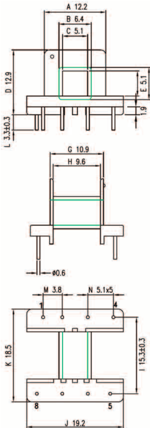
ТPI-0501908(H) - каркас 1 секция 8 выводов (EI-19-5-8PIN)
