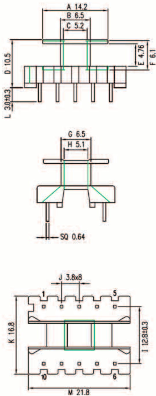
TPI-0501861(V) - каркас 1 секция 10 выводов (EI-186-10PIN)
