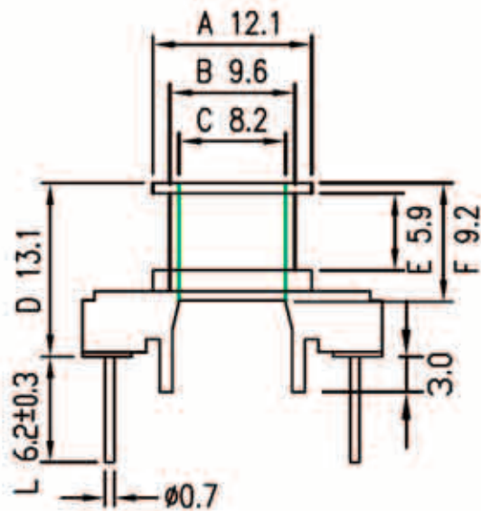
ТП-0501905(V) - каркас 1 секция 6 выводов (EI-19-8-2-6PIN)
