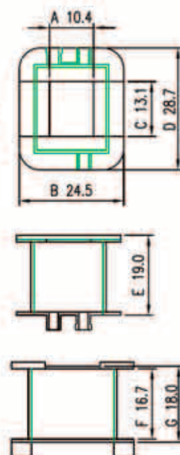
TPI-0503502(V) каркас 1 секция (EI-35-13B)
