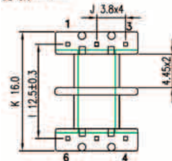
TPI-0501611(H) - каркас 1 секция 6 выводов (EE-16-6PIN-1SEC)
