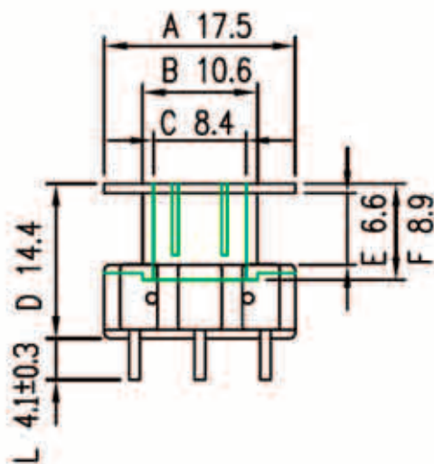
TPI-0502807(V) - каркас 1 секция 6 выводов (EI-28-12.5-2-6PIN)
