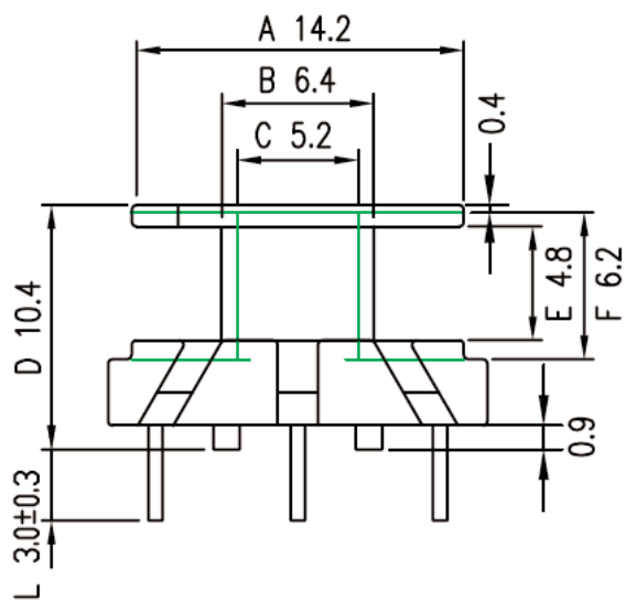
TPI-0501862(V) - каркас 1 секция 6 выводов (EI-186-6PIN)
