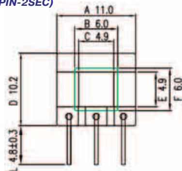
TPI-0501607(V) - каркас 2 секции 6 выводов (EE-16-6PIN-2SEC)
