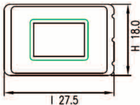
TPI-0502812(V) - каркас 1 секция (EI-28-12C)
