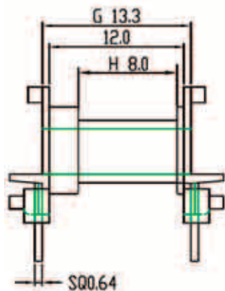
TPI-0501614(H) - каркас 1 секция 4 вывода (EE-16-4-4PIN)
