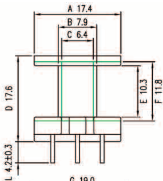
TPI-0502401(V) - каркас 1 секция 6 выводов (EI-24-7-6PIN)
