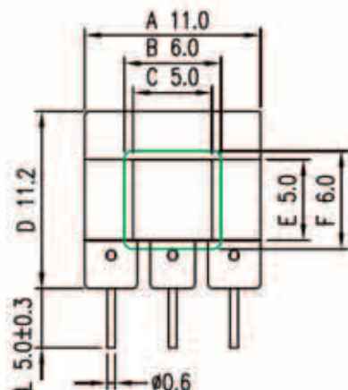
TPI-0501608(H) - каркас 2 секции 6 выводов (EE-16-6PIN-2SEC)
