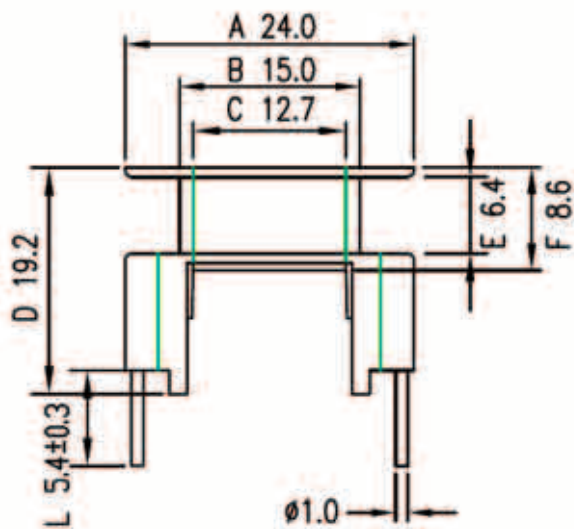
TPI-0502810(V) - каркас 1 секция 6 выводов (EI-28-12-6PIN)
