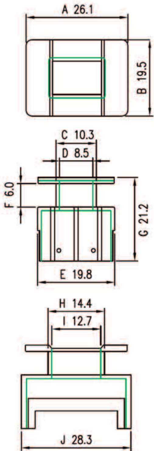
TPI-0502806-1(V) - каркас 1/2 секции (EI-28-12.5C)
