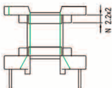
TPI-0502405(V) - каркас 1 секция 8 выводов (EI-24-7-8PIN)
