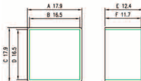
TPI-0501612 - крышка (EE-16-CASE)
